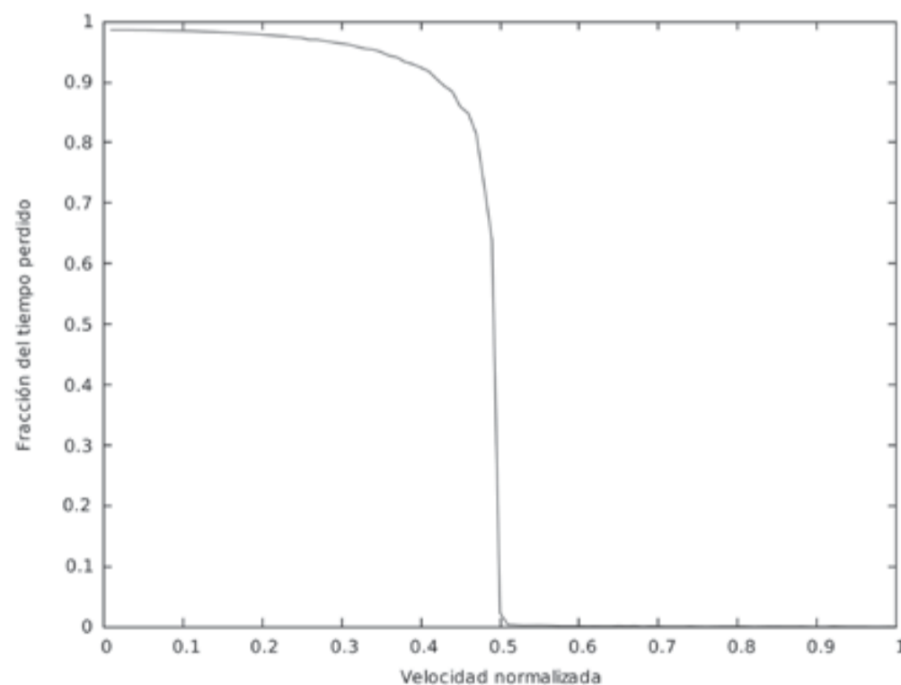
Figura 4. Tiempo perdido por los autos en embotellamientos viales como función de la velocidad máxima permitida.
