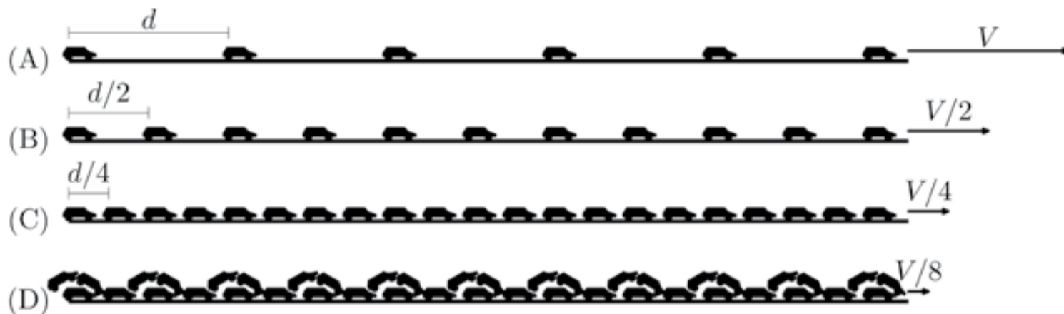
Figura 3. (A) Conjunto de autos espaciados una distancia d entre sí, circulando con un flujo dado f sobre cierta calle a cierta velocidad V . (B) Conjunto similar de vehículos circulando a una velocidad menor V/2 pero espaciados una distancia menor d/2 , por lo cual su densidad es más alta y su flujo f es el mismo que en la parte superior. (C) Conjunto de autos viajando aún más lentamente, espaciados una distancia aún menor y con una densidad aún mayor, pero con el mismo flujo. (D) A una velocidad demasiado baja el sistema colapsa y no se puede conservar el flujo, pues para ello los autos tendrían que encimarse unos sobre otros.
